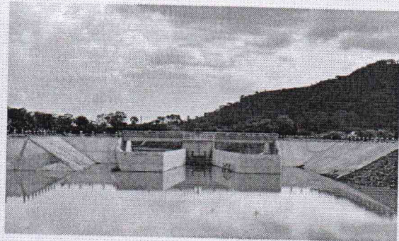
( รูปงานอาคารบังคับน้ำคลองห้วยทราย ตำบลเขาพระ อำเภอเมือง จังหวัดนครนายก )
