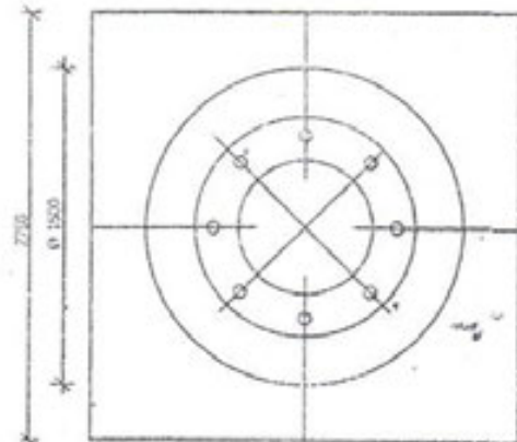
แปลนฐานรากชนิดไม่ตอกเข็ม
