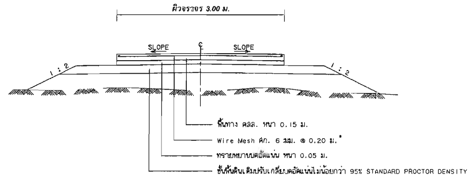
รูปตัดถนน คลล. NOT TO SCALE
