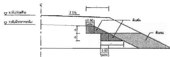
รูปตัดการก่อสร้างลาดคันทางบนถนนเดิม งานตัดได้แก่(งานตัดดิน,งานตัดหินผุ,งานตัดหินแข็งและงานตัดอื่นๆ)
