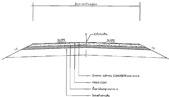
รูปตัดแสดงความกว้างและหน้าผิวจราจร
