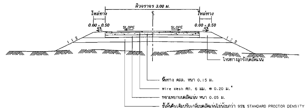
รูปตัดถนน คล.ล. NOT TO SCALE
