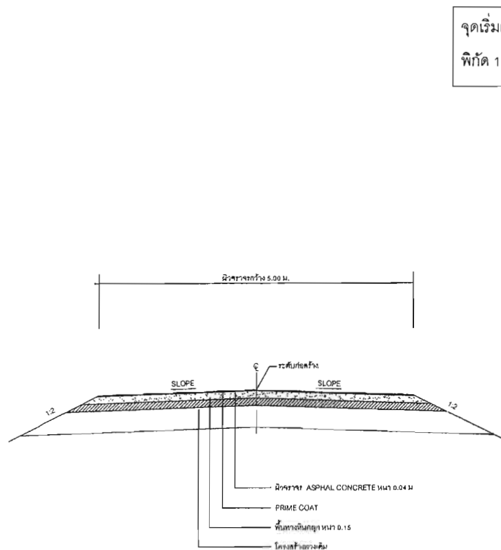
รูปตัดแสดงความกว้างและหน้าผิวจราจร
