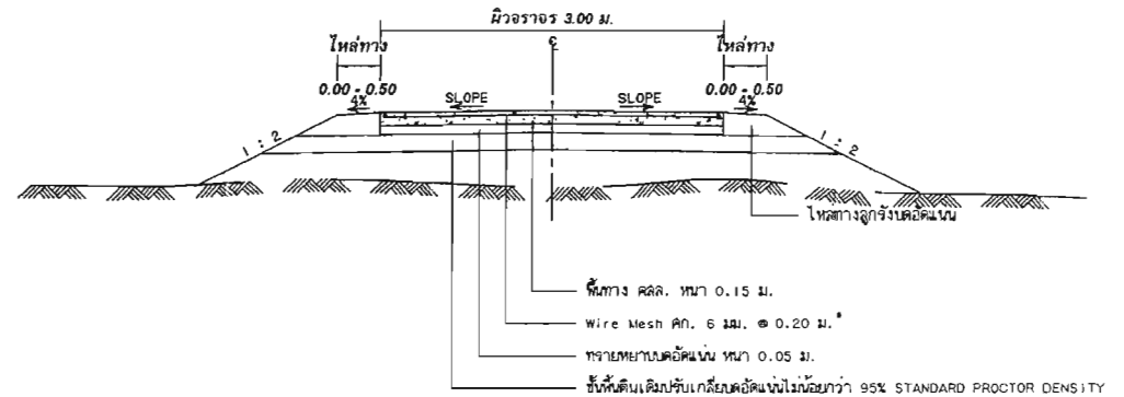
รูปตัดถนน คลส. NOT TO SCALE
